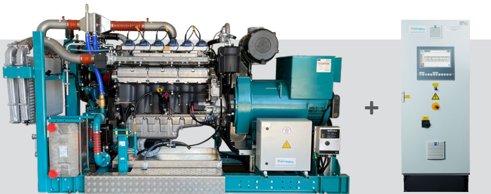
Umrüsten inkl. Schaltschrank mit Touchpanel.
